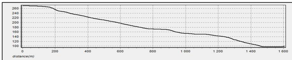
Fig. 102 Profil topografic longitudinal prin vârful Poiana, la sud de Crăciun
