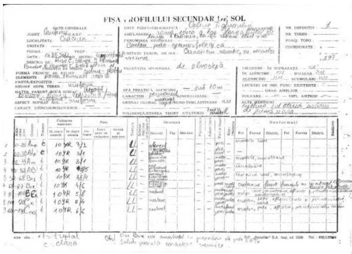
Fig. 8 Fișa profilului de sol
