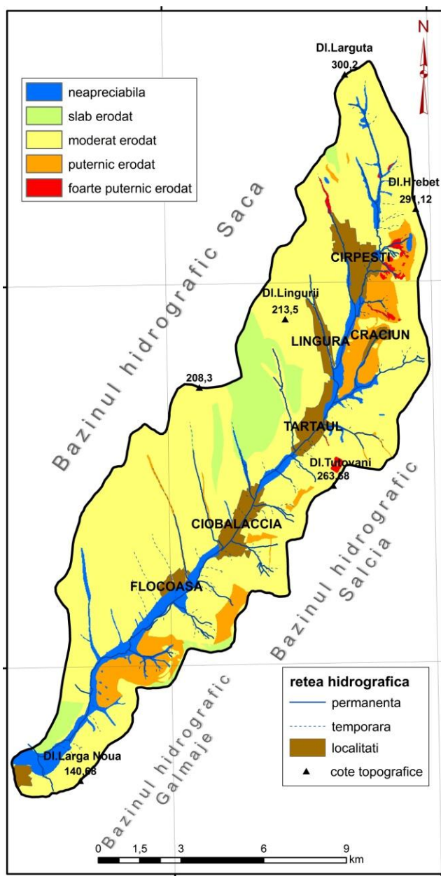
Fig. 128 Harta erodabilității solurilor (după Moțoc și colab., 1975)
