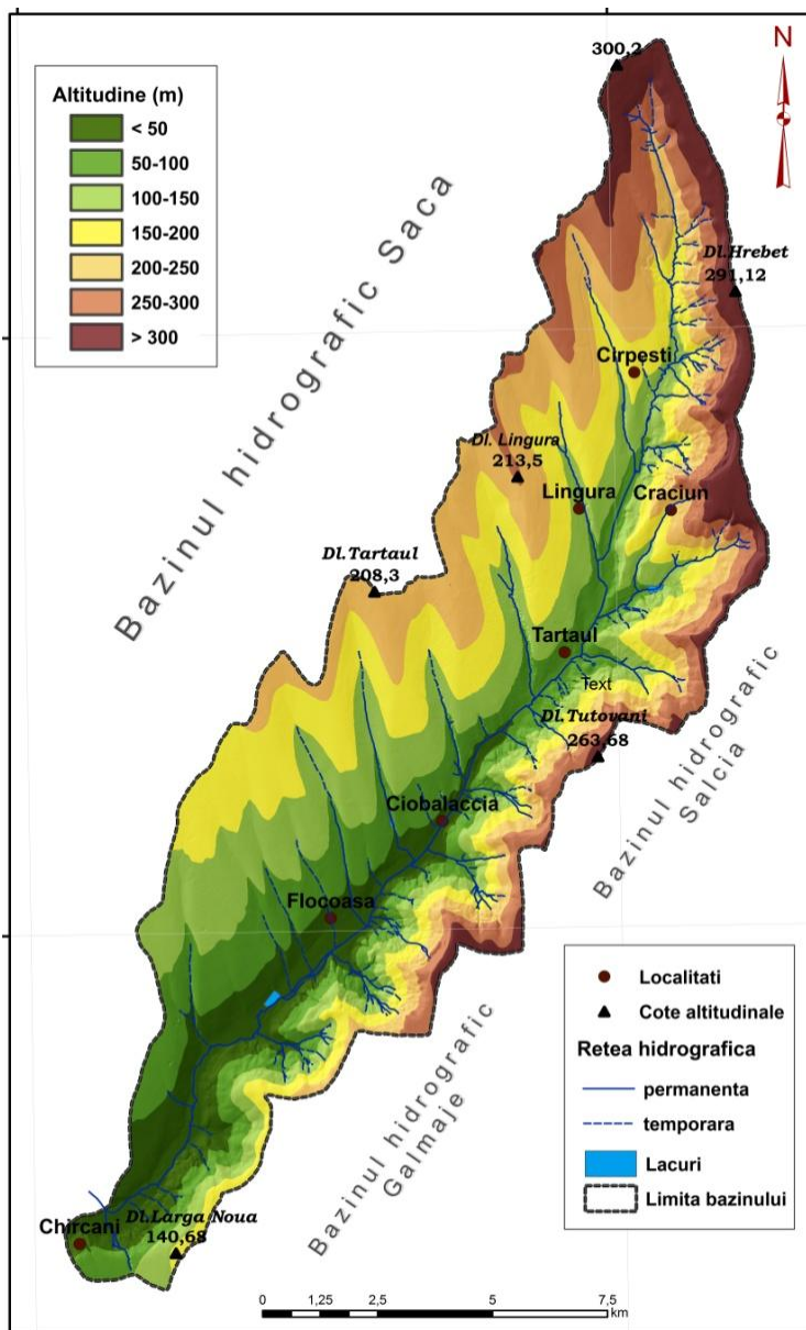
Fig. 36 Harta hipsometrică din bazinul hidrografic Larga
