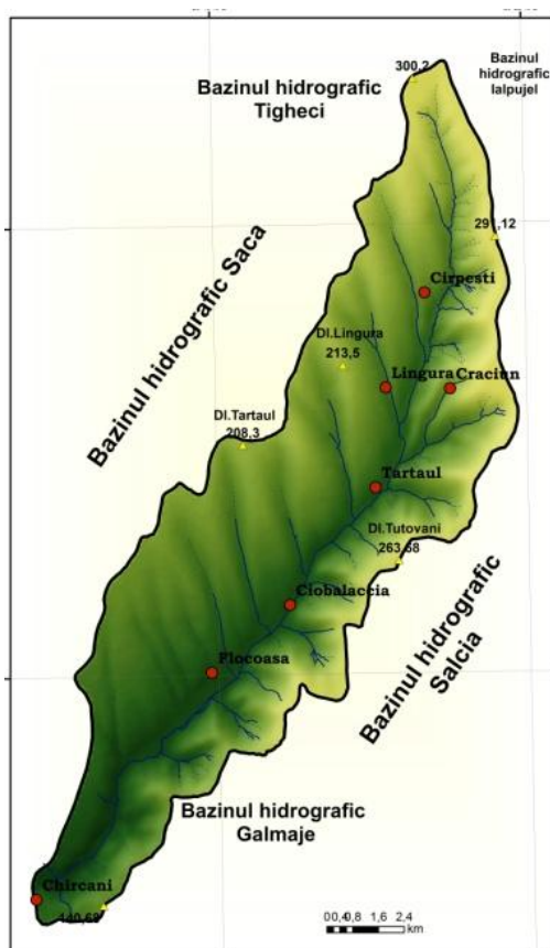
Fig. 2 Limitele hidrografice ale bazinului Larga
