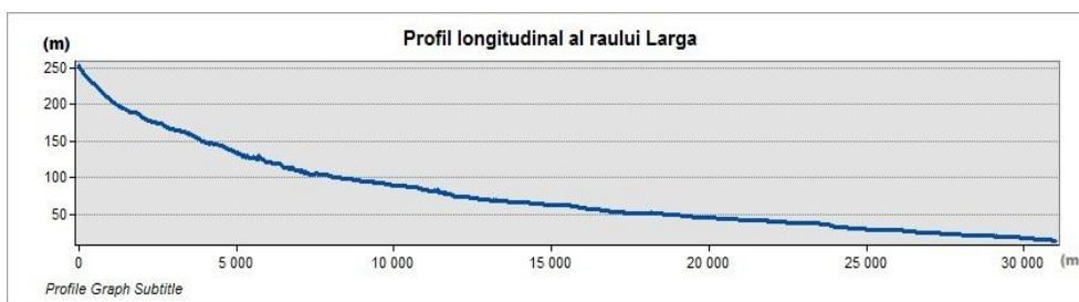
Fig. 24 Profilul longitudinal al râului Larga
