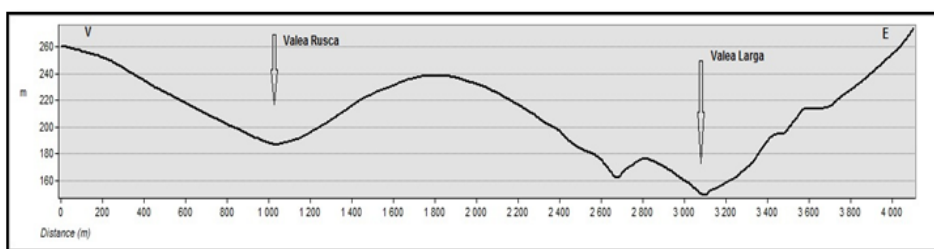
Fig. 31 Profil transversal pe direcție V-E în bazinul superior al Largăi
