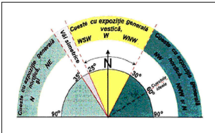
Fig. 56. Schema domeniilor potențiale de răspândire a cuestelor (Ioniță, 1998)
