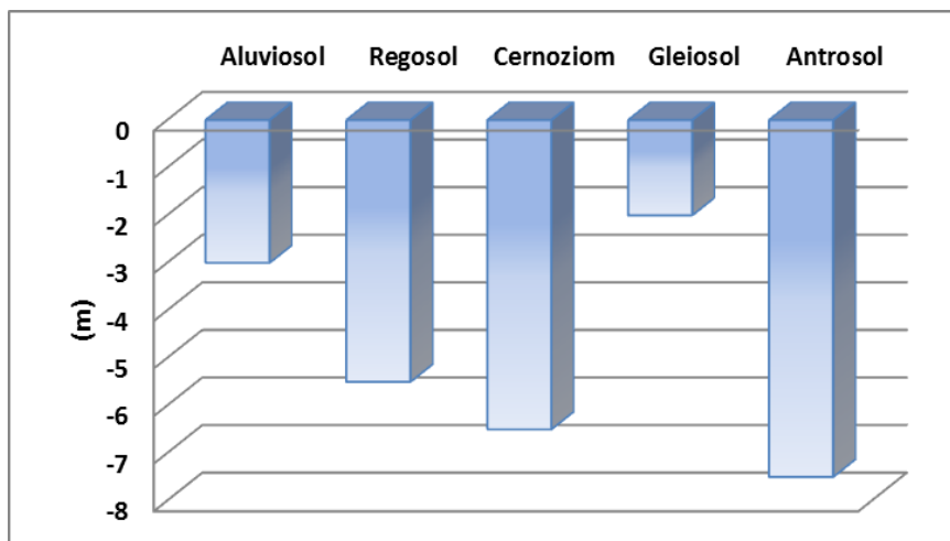
Fig. 113 Adâncimea medie de apariție a apei freatice pe tipuri de sol
